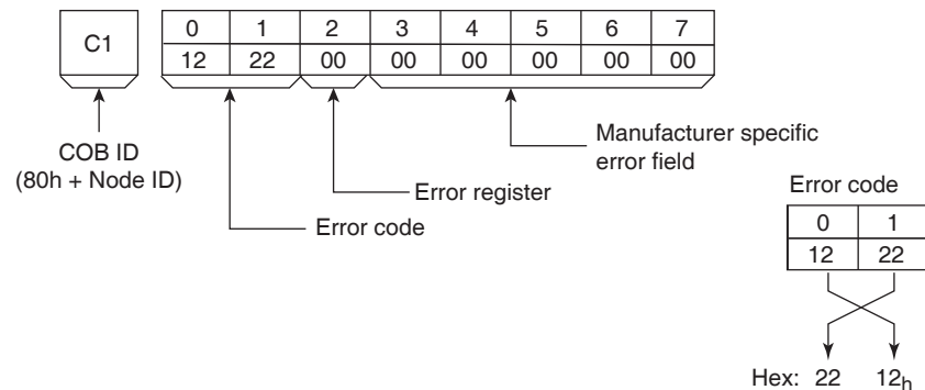
Figure 1.27 - EMCY Message
