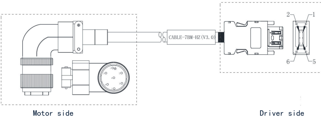
Motor cable pin
