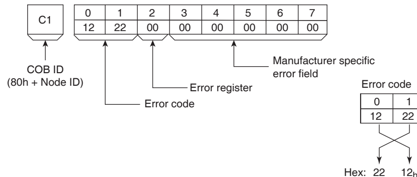
Figure 1.27 - EMCY Message
