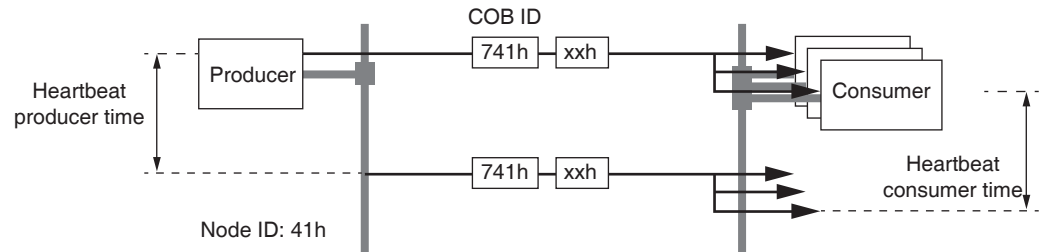
Figure 1.33 - «Heartbeat» Monitoring
